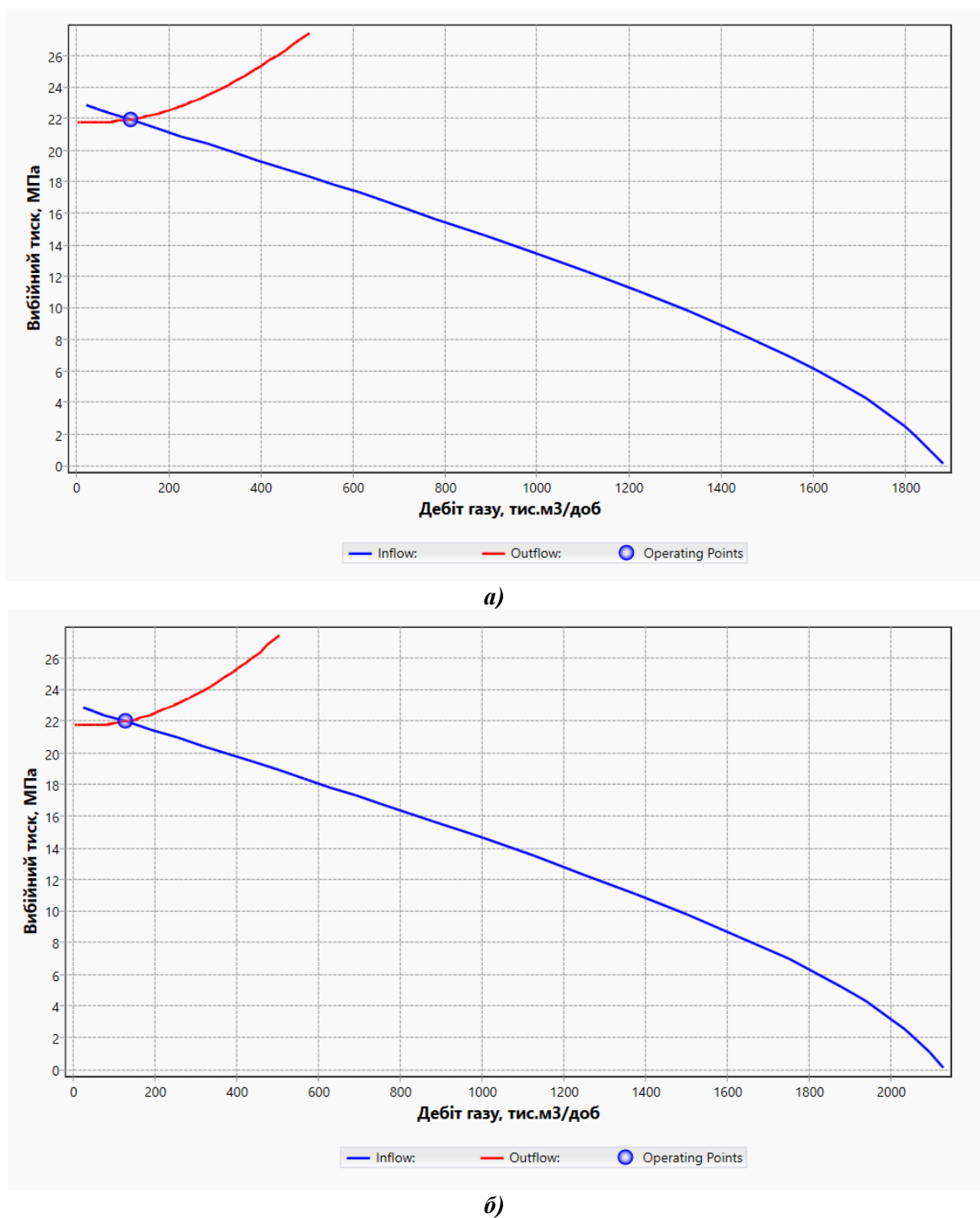
Рисунок 1 – Вузловий аналіз роботи газової свердловини з гравійним фільтром у перфорованій експлуатаційній колонії для діаметрів фільтра-каркасу 0,0603 м (а) та 0,073 м (б) за кількості перфораційних каналів 20 на один метр розкритої товщини пласта та їх діаметру 11 мм
