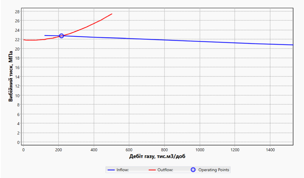
Рисунок 5 – Вузловий аналіз роботи модельної газової свердловини з гравійним фільтром у відкритому стовбурі
